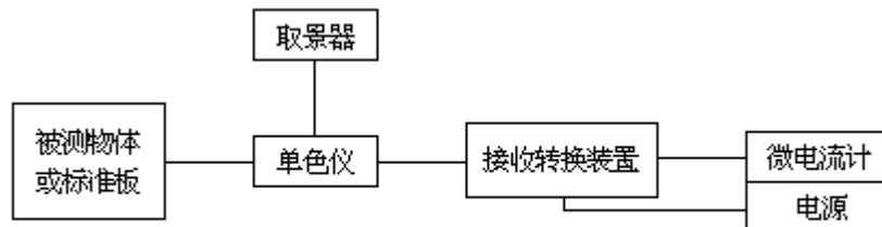
图 2-17 棱镜式野外分光光度计
