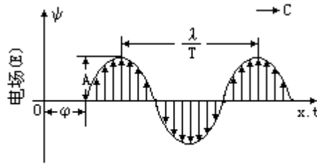
图 2-1 波函数图解
