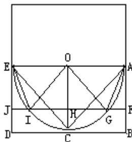
图4 正弦求弧背术（用圆内积）
