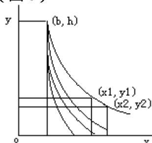
图5 对数合尖锥曲线
