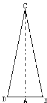
图 38 一光行差
