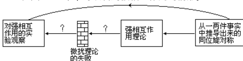
图 11.2 从 20 世纪 30 年代到 70 年代初强相互作用研究的图景。
