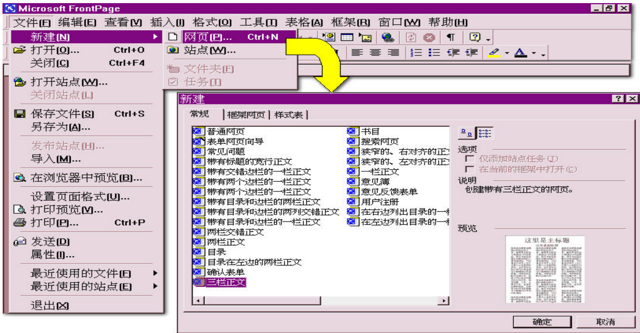
图 1.26 创建网页
