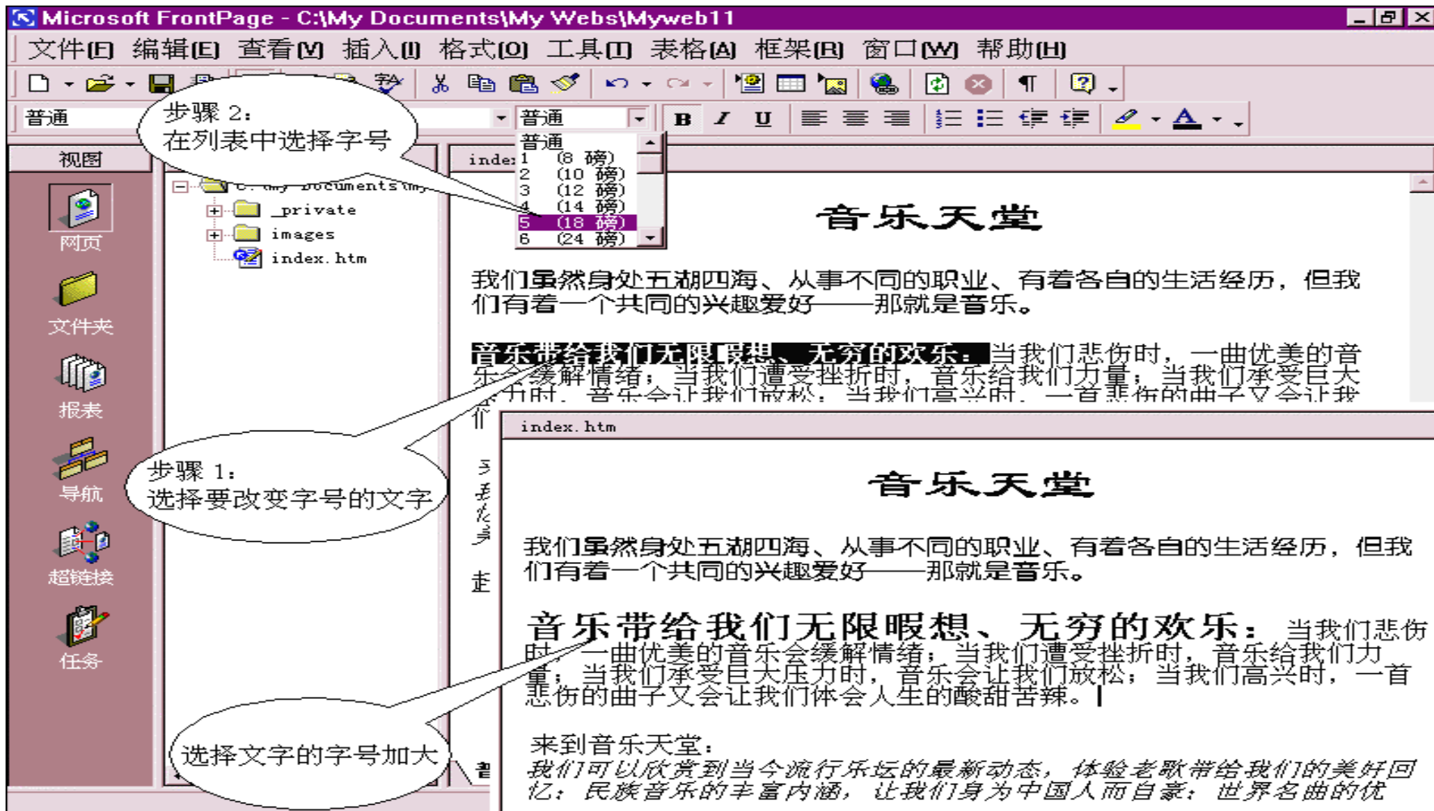
图 3.16 设置字号
