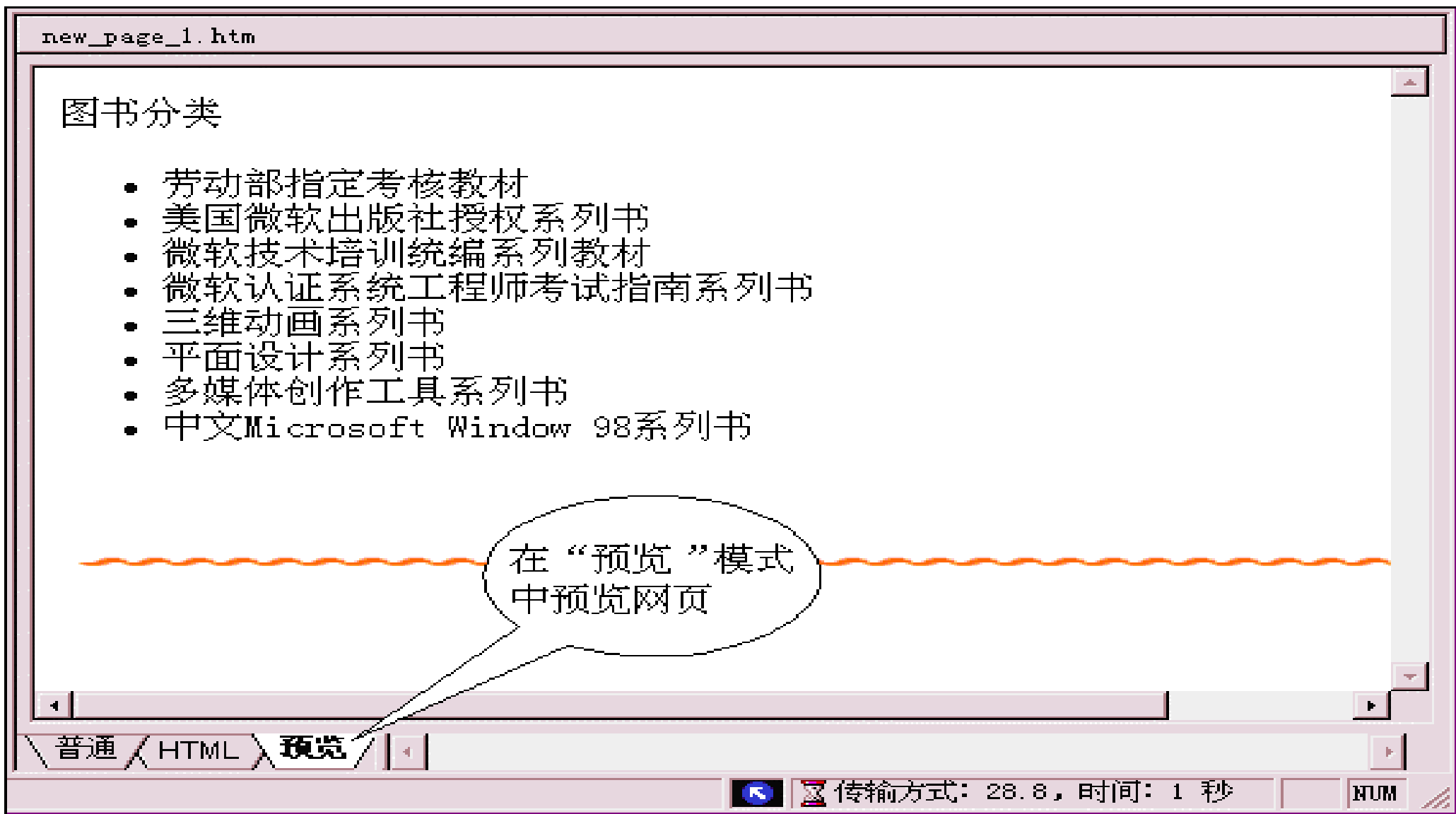
图 3.62 预览模式
