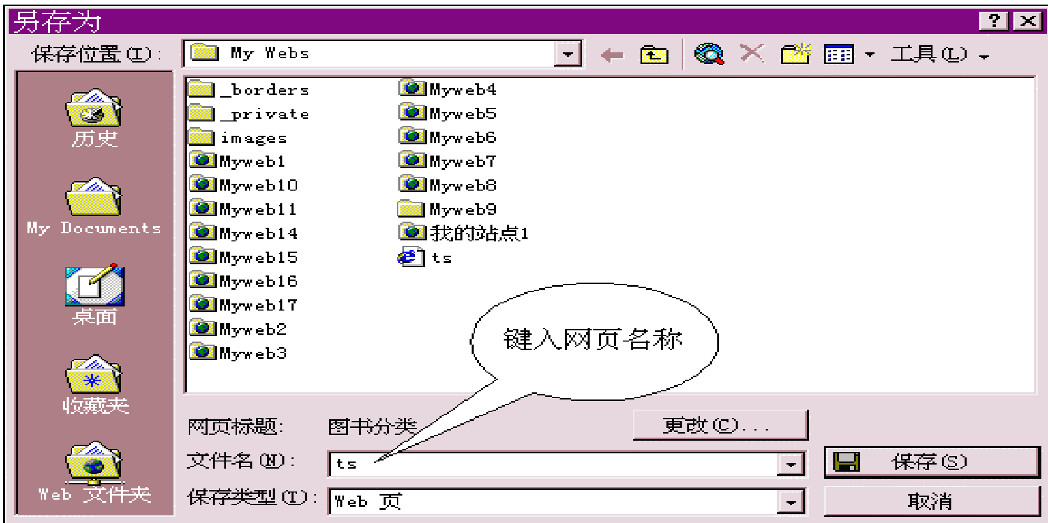
图 3.65 保存网页
