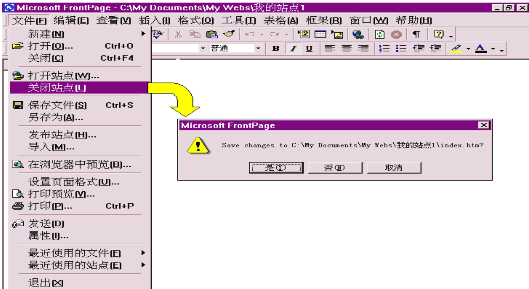
图 1.51 关闭站点
