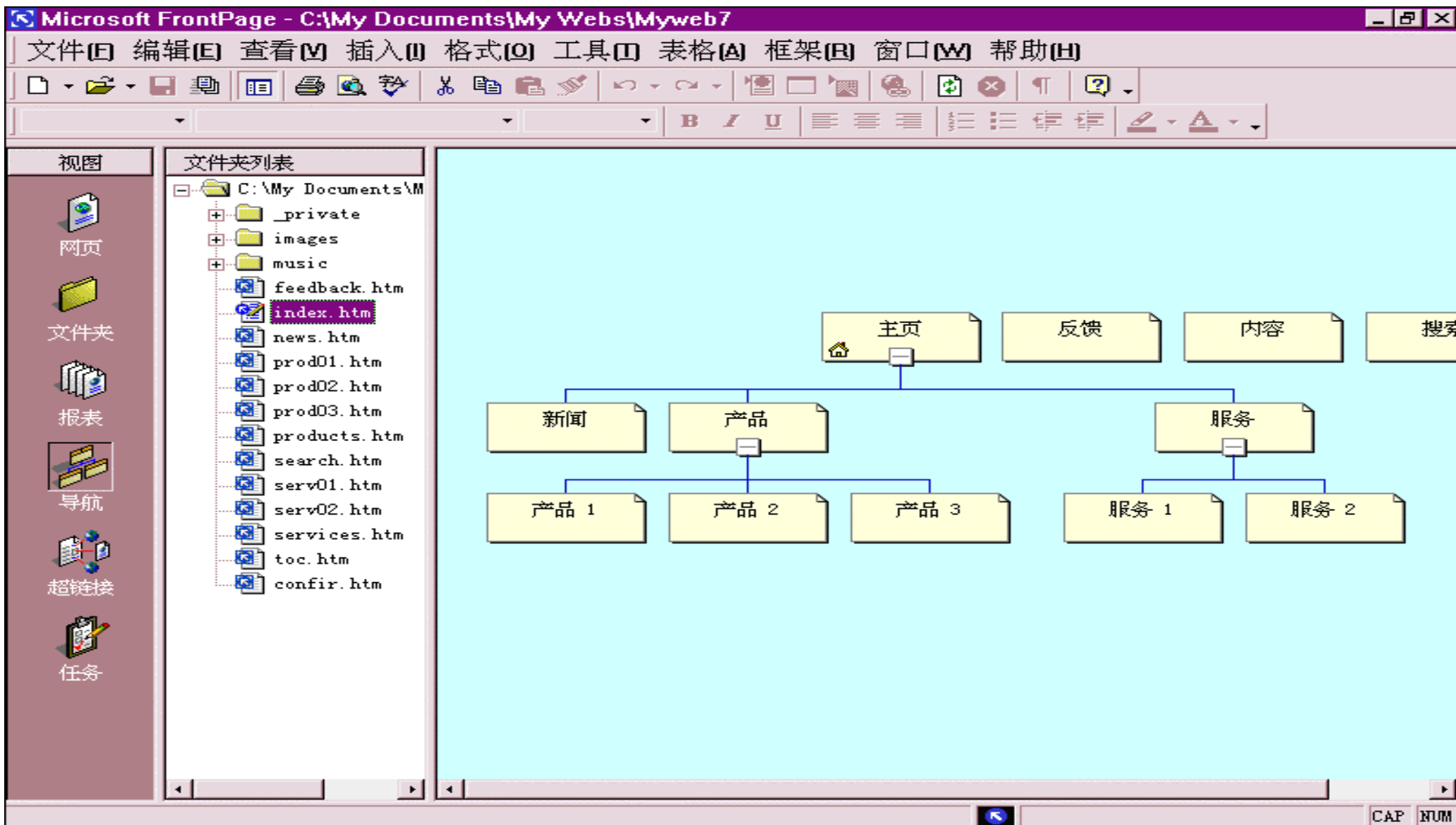
图 1.39 导航结构图
