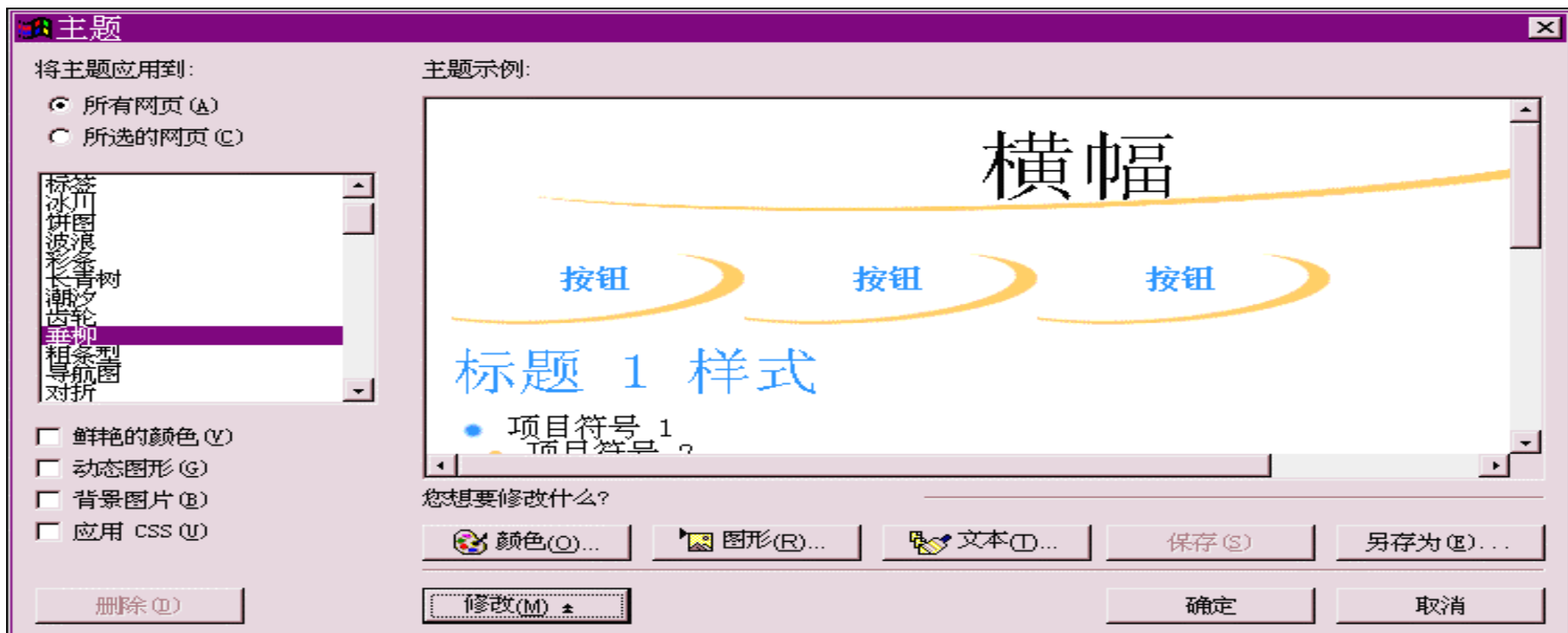
图 1.18 FrontPage 的主题
