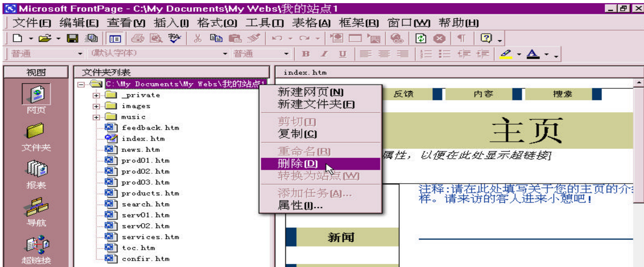
图 1.45 删除站点
