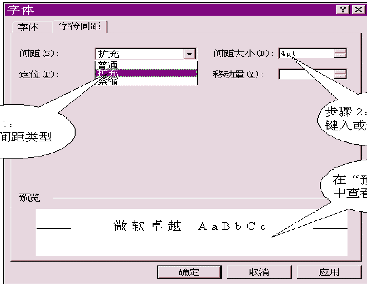
图 3.20 设置字符间距
