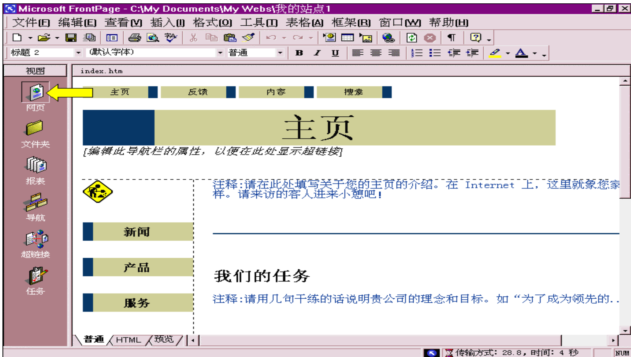
图 1.52 “网页”视图
