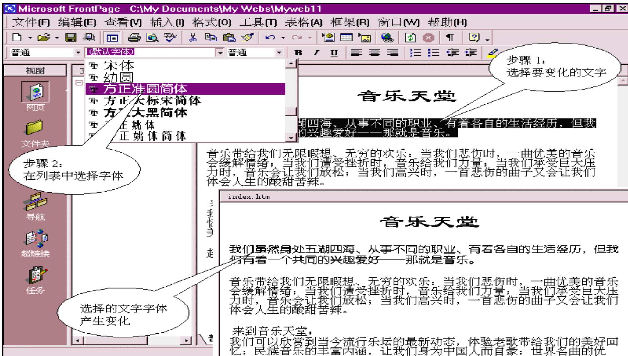
图 3.14 设置字体
