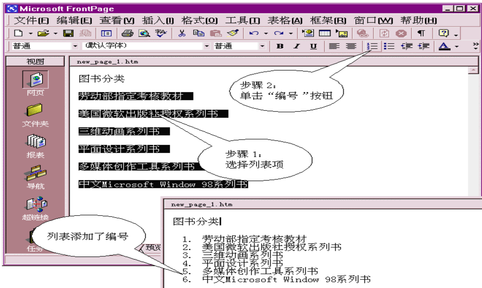
图 3.31 添加编号
