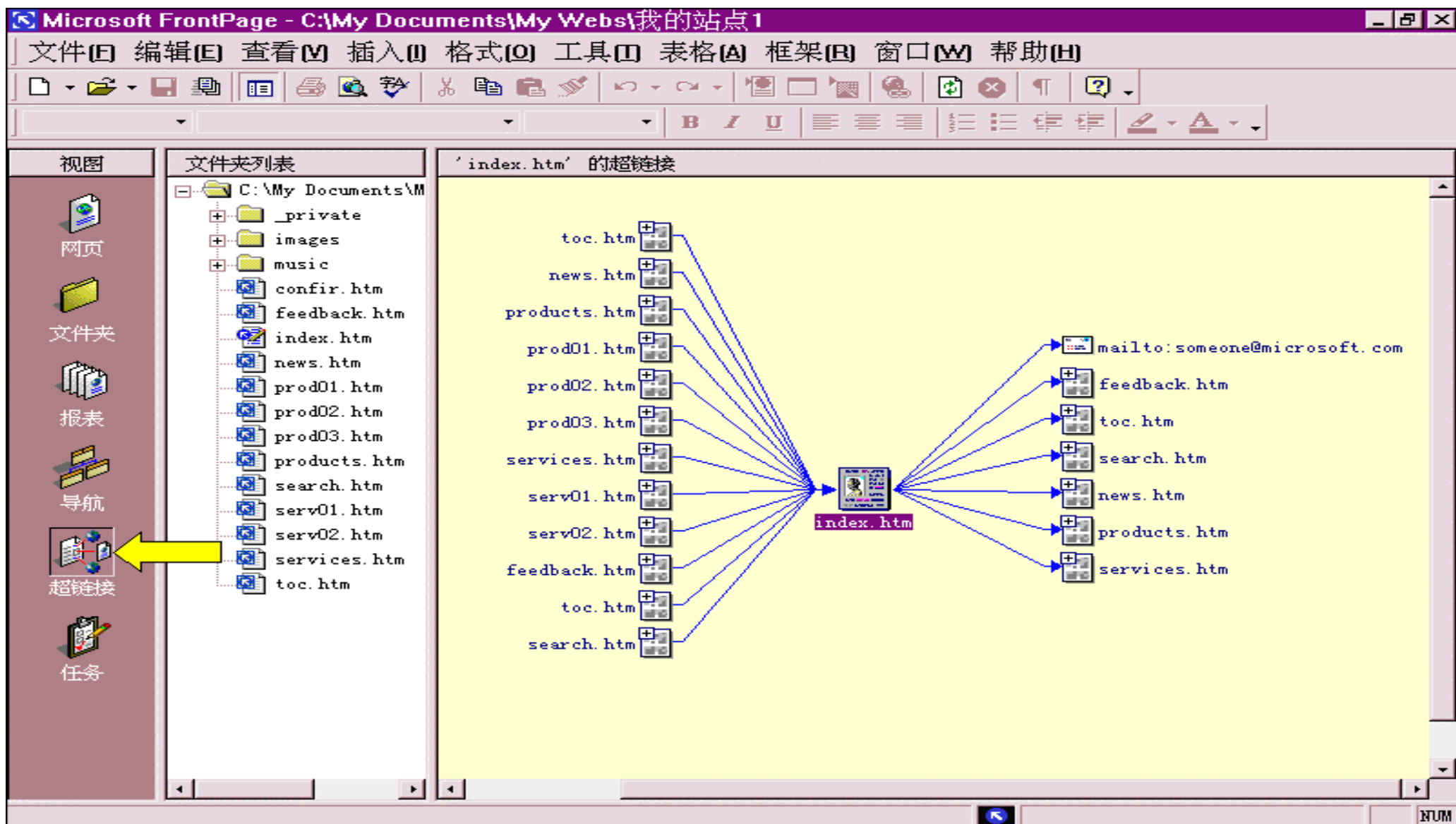
图 1.56 “超链接”视图
