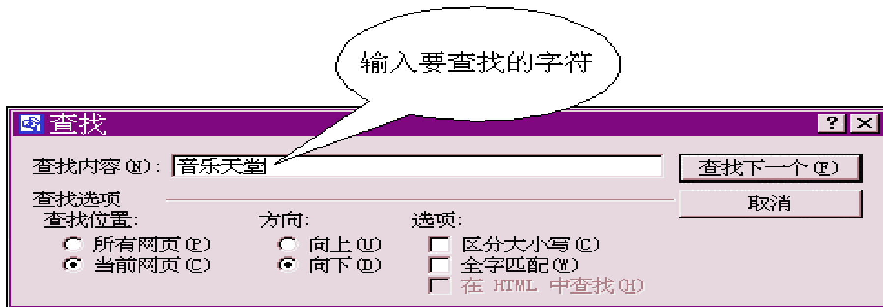
图 3.11 查找字符串
