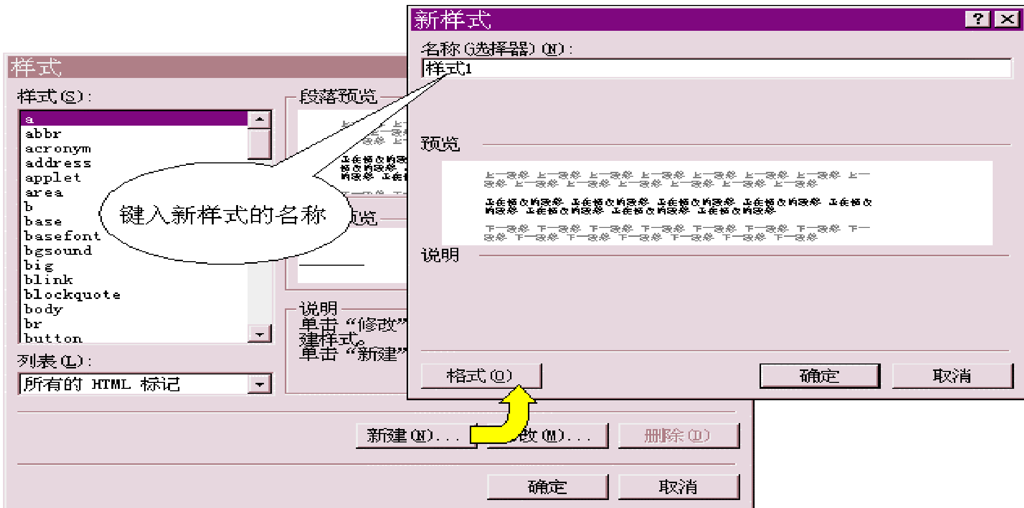
图 3.24 建立新样式
