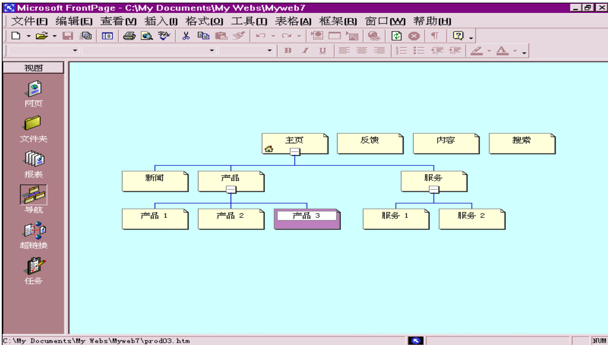
图 1.22 站点结构
