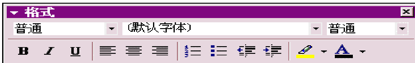
图 3.13 “格式”工具栏
