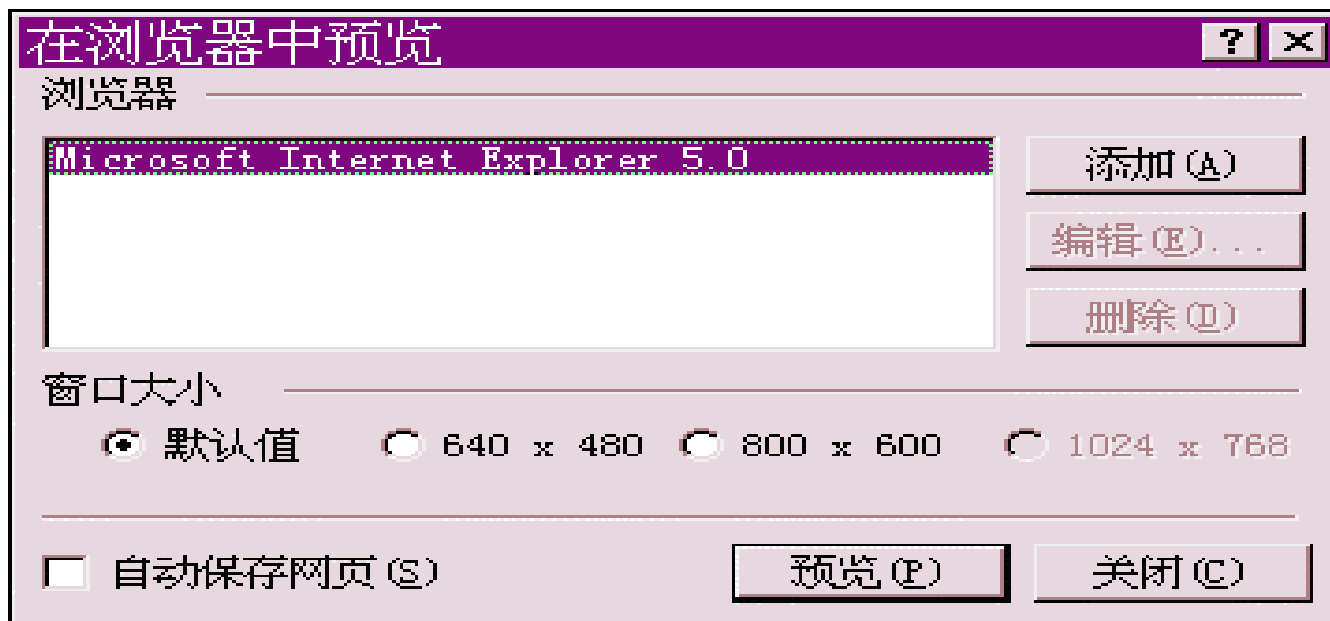
图 3.63 选择浏览器
