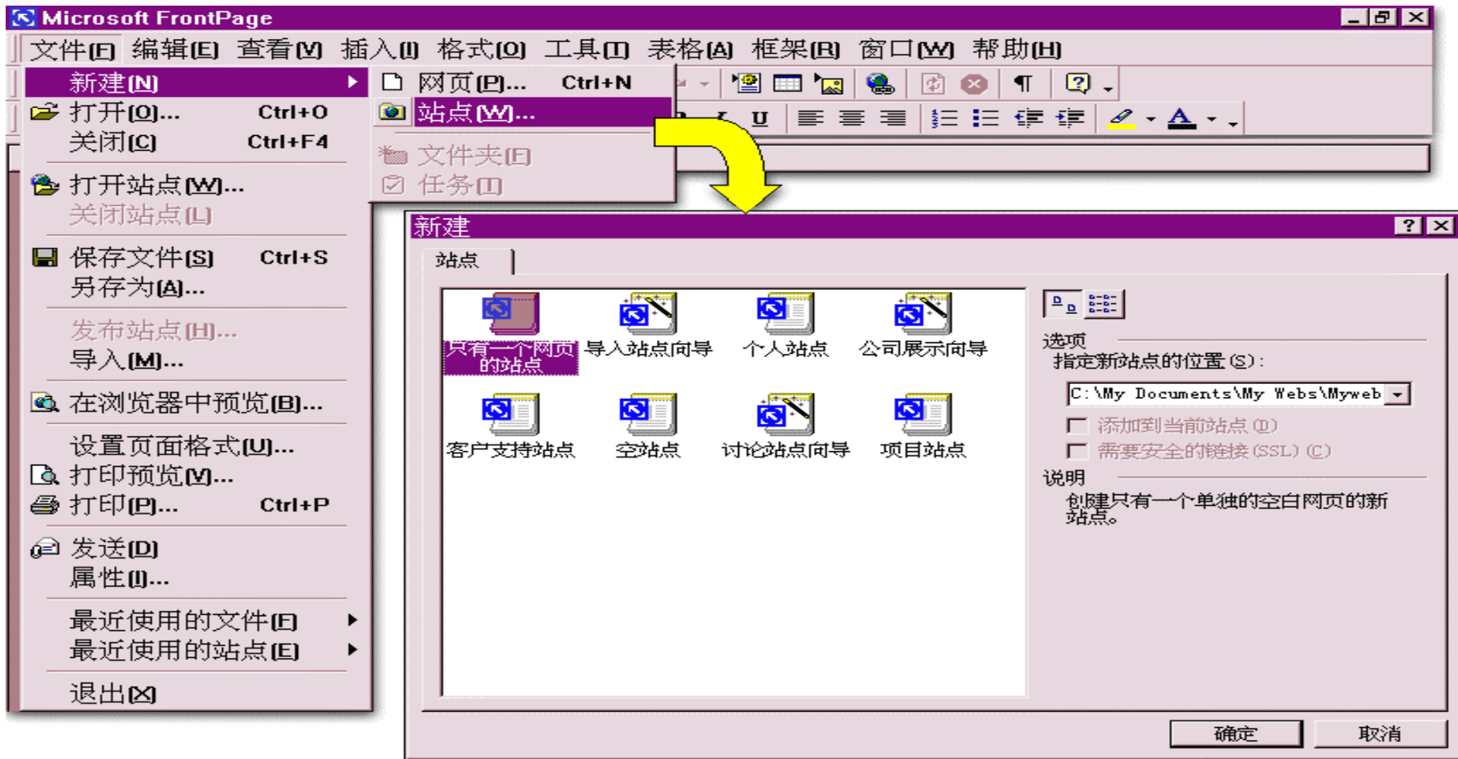
图 1.25 “新建”对话框
