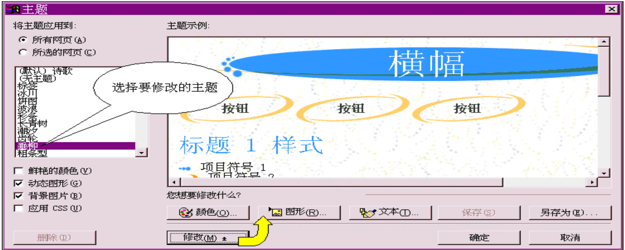
图 3.54 修改选项
