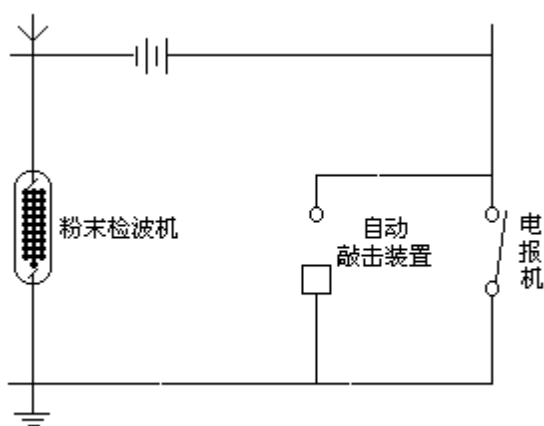
马可尼的收报装置
