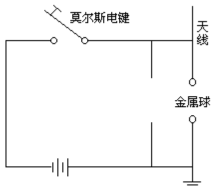
马可尼的发报装置
